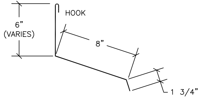
Endwall
