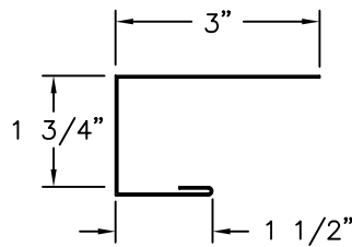
C-METAL
