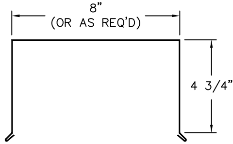
PARAPET CAP
