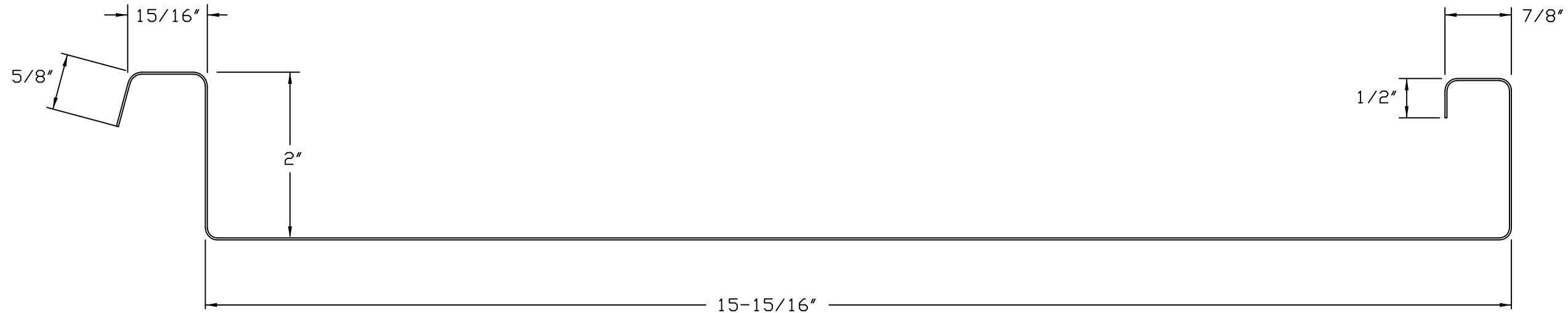
SPANSEAM
